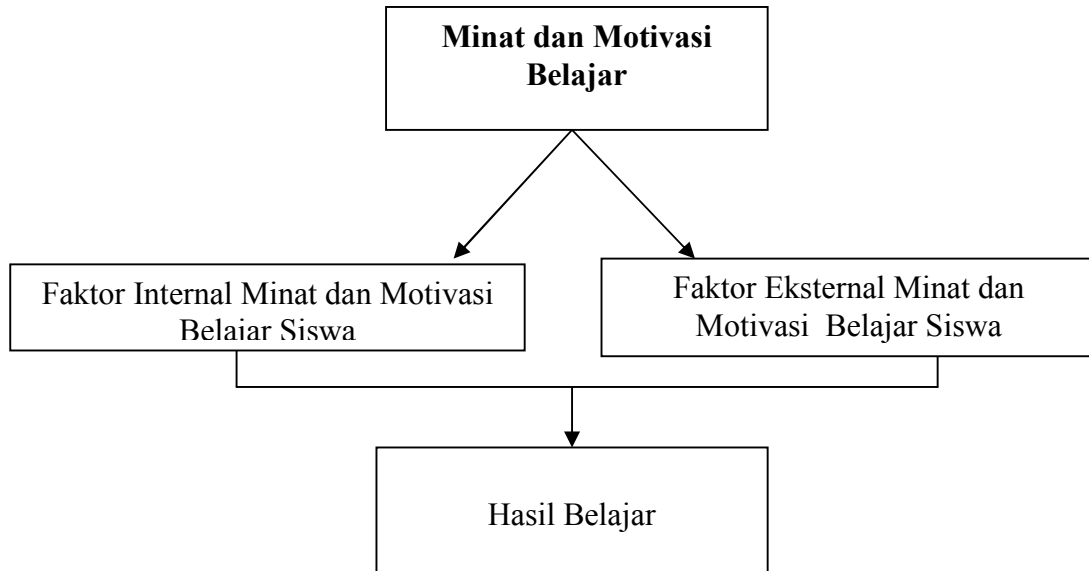
Gambar 1 Kerangka Berpikir
