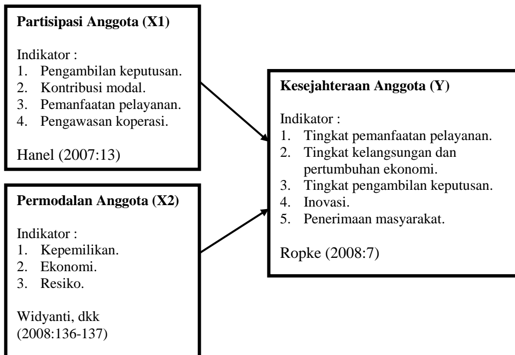
Gambar 1 Kerangka Berpikir
