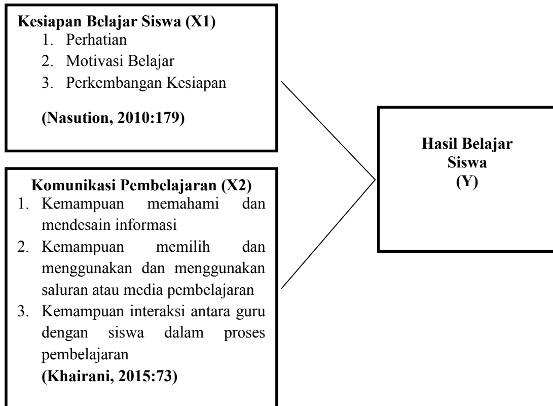
Gambar 1 Kerangka Berpikir
