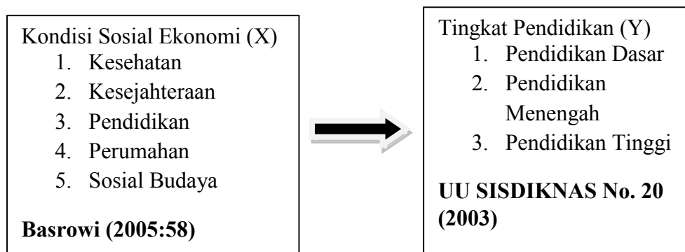
Gambar 1 Kerangka Berpikir
